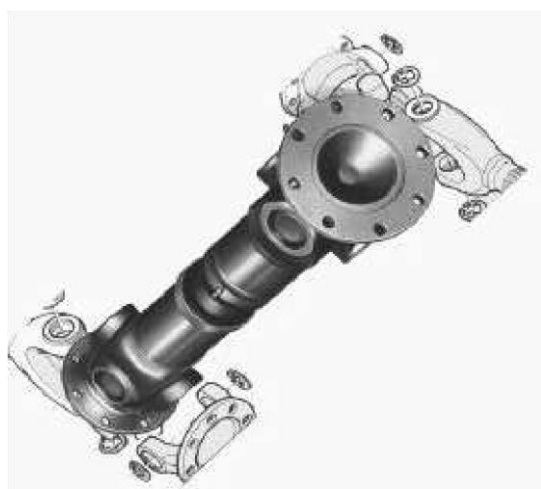
Juntas telescópicas de precisión
